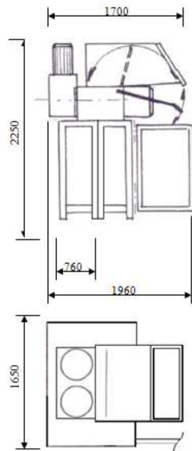
Dimensions
